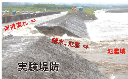
実物大規模の堤防決壊実験
