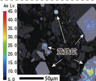
電子顕微鏡で見た黄鉄鉱中の ヒ素(As)の濃度分布
