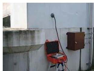
頭首工における補修・補強工法の耐久性調査
