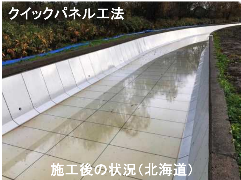
施工後の状況(北海道)
