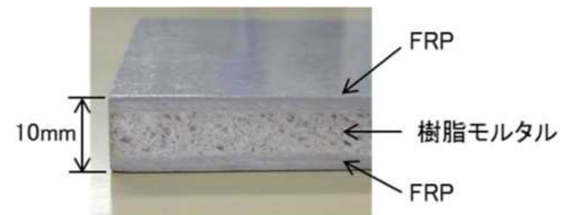
FRPM板の構造
