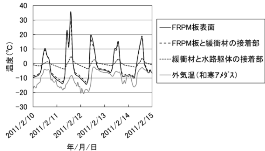
冬期間の試験施工区間の温度変化
