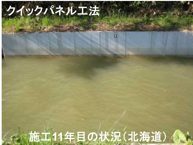
水路更生工法
