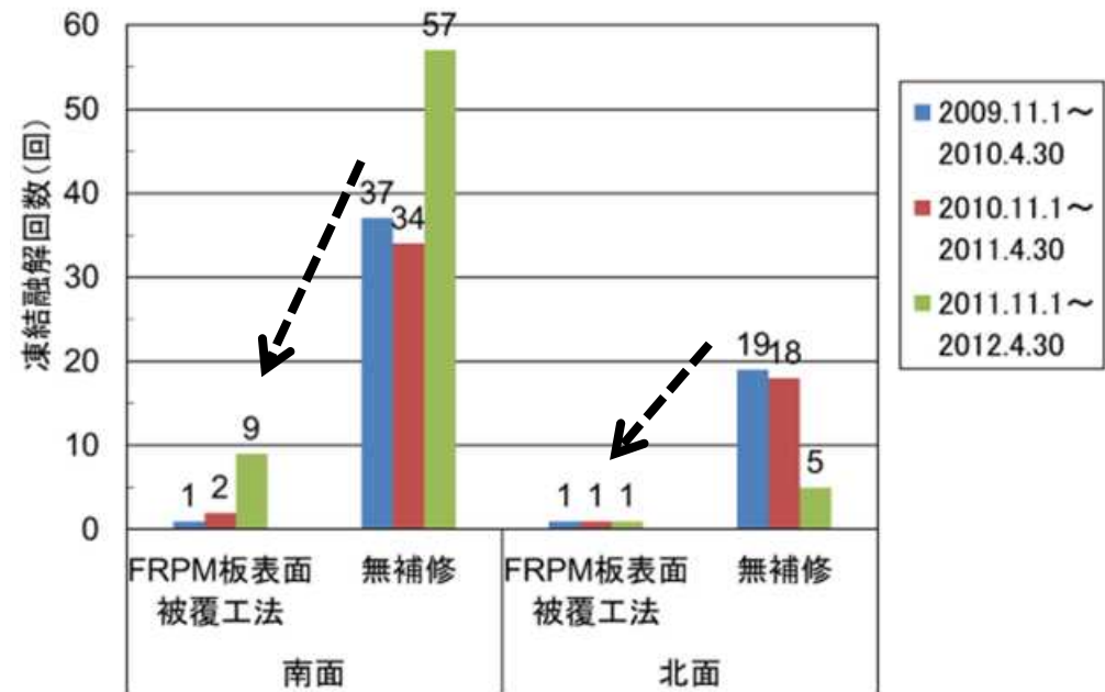
FRPM板で補修した場合と無補修の場合の水路躯体コンクリートの凍結融解回数※ 10
