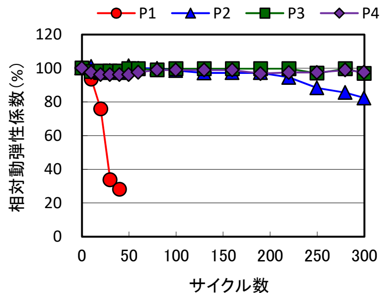
一次共鳴振動数(たわみ振動)
