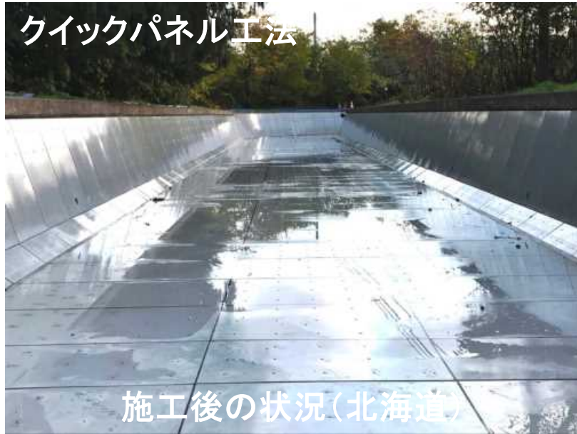
クイックパネル工法
