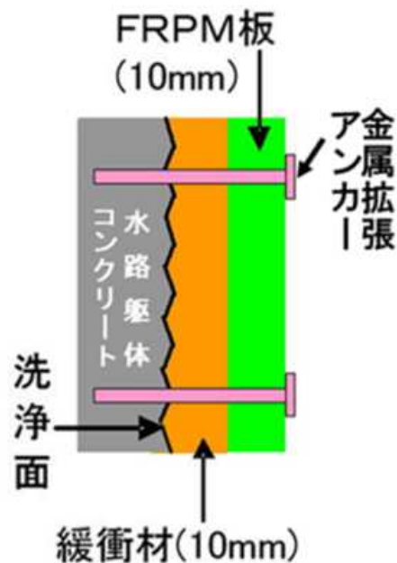
FRPM板ライニング工法「クイックパネル工法」 断面概要
